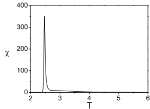
(d) 16^3 , \Delta_0 = 2.0 , seed: 1050
